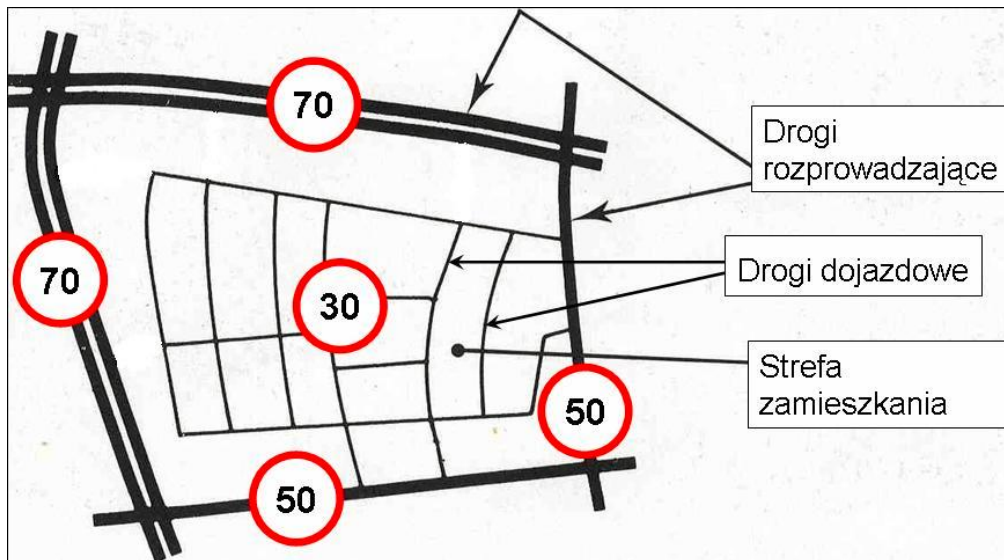
Rysunek 14-5 Strefowanie prędkości w mieście
