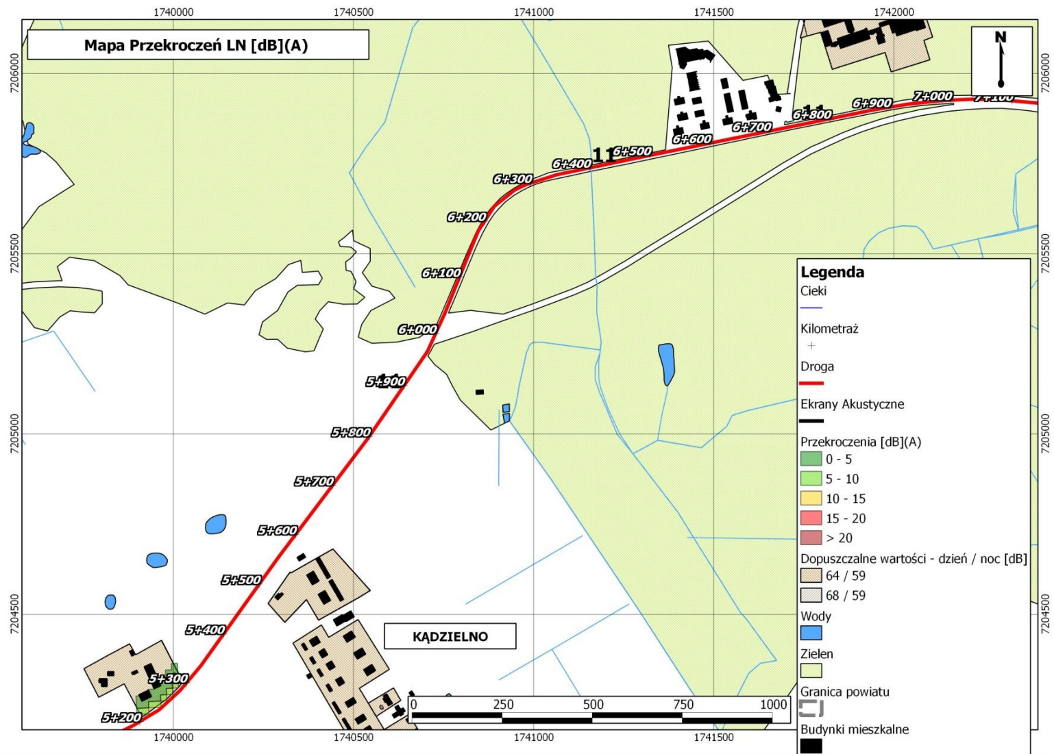
Rysunek 1-82 Przekroczenia dopuszczalnych poziomów hałasu drogowego – drogi krajowe - Kądzierzno - wskaźnik LN
