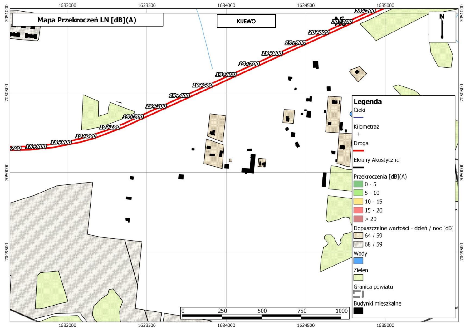
Rysunek 1-118 Przekroczenia dopuszczalnych poziomów hałasu drogowego – drogi krajowe - Kijewo - wskaźnik LN
