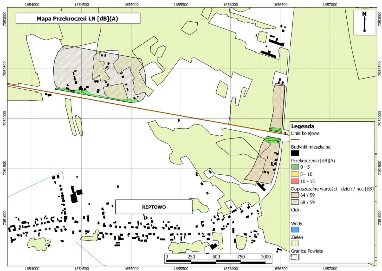
Rysunek 3-8 Przekroczenia dopuszczalnych poziomów hałasu kolejowego - Reptowo - wskaźnik LN
