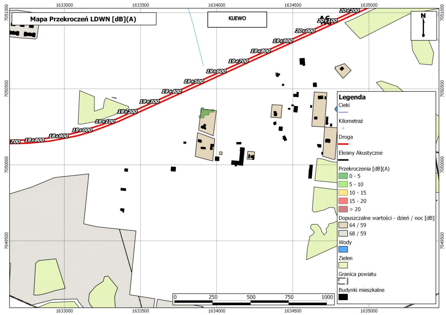
Rysunek 1-117 Przekroczenia dopuszczalnych poziomów hałasu drogowego – drogi krajowe - Kijewo - wskaźnik LDWN
