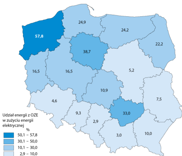
Rysunek 19. Udział produkcji energii elektrycznej z OZE w jej zużyciu ogółem w % według województw w 2018 r.
