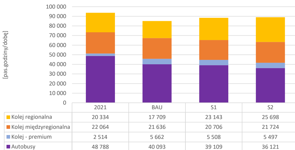
Rysunek 4.10 Zestawienie dobowej pracy przewozowej wyrażona w pojazdgodzinach w transporcie zbiorowym dla poszczególnych scenariuszy Źródło: opracowanie własne
