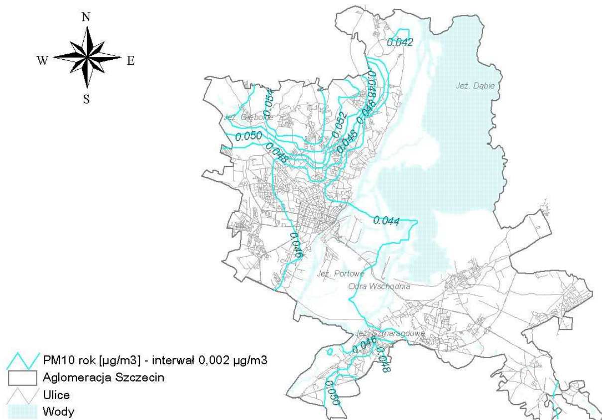
Rysunek 10 Stężenia pyłu zawieszonego PM 10 o okresie uśredniania wyników rok kalendarzowy na terenie aglomeracji Szczecin, pochodzące od emitorów punktowych z Niemiec w 2006 r
