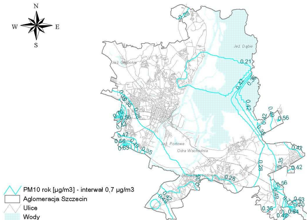
Rysunek 14 Stężenia pyłu zawieszonego PM_{10} o okresie uśredniania wyników pomiarów rok kalendarzowy na terenie aglomeracji Szczecin, pochodzące od emitorów liniowych zlokalizowanych w pasie 30 km wokół aglomeracji w 2006 r
