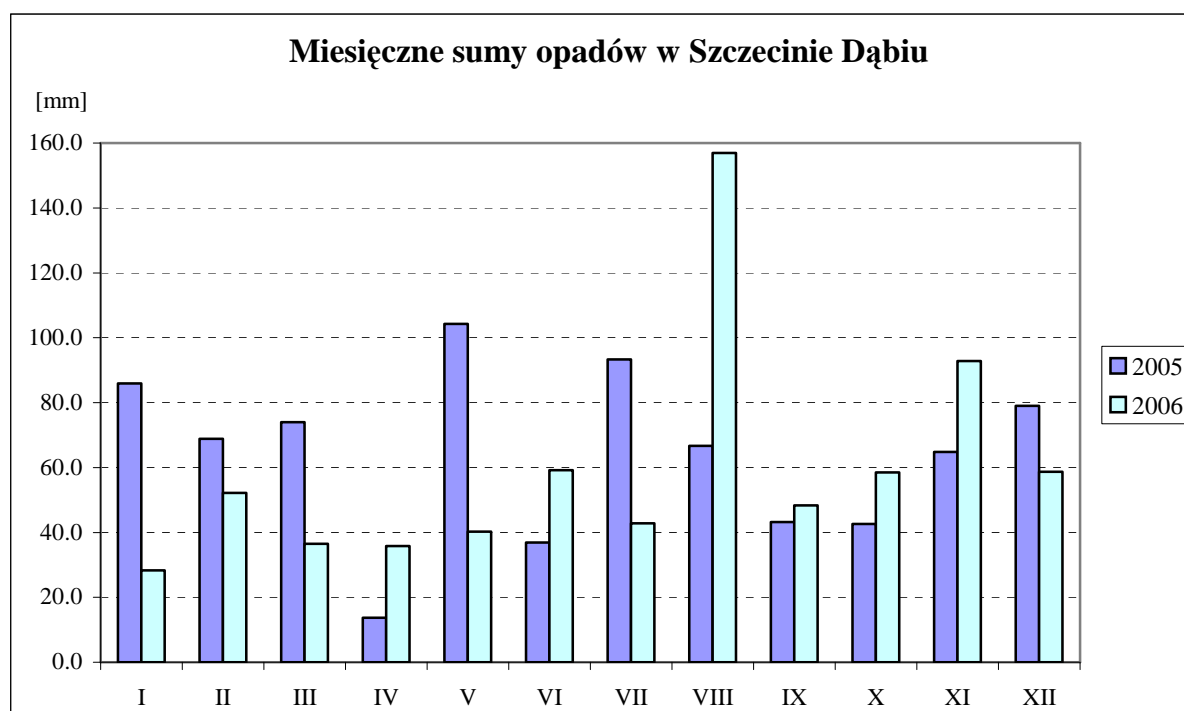
Rysunek 2 Miesięczne sumy opadów w Szczecinie Dąbie w latach 2005 i 2006.
