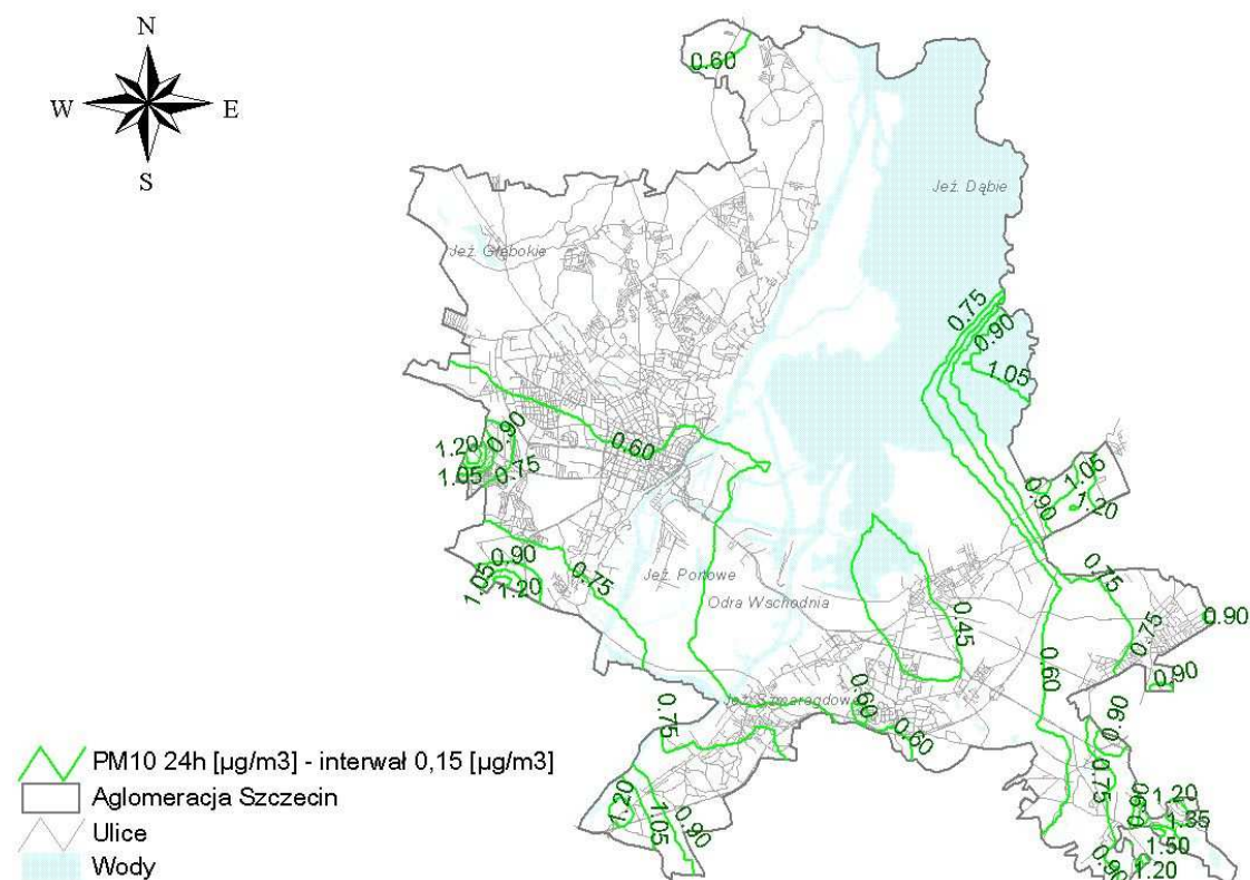
Rysunek 13 Stężenia pyłu zawieszonego PM_{10} o okresie uśredniania wyników pomiarów 24 godziny na terenie aglomeracji Szczecin pochodzące od emitorów liniowych zlokalizowanych w pasie 30 km od aglomeracji w 2006 r.
