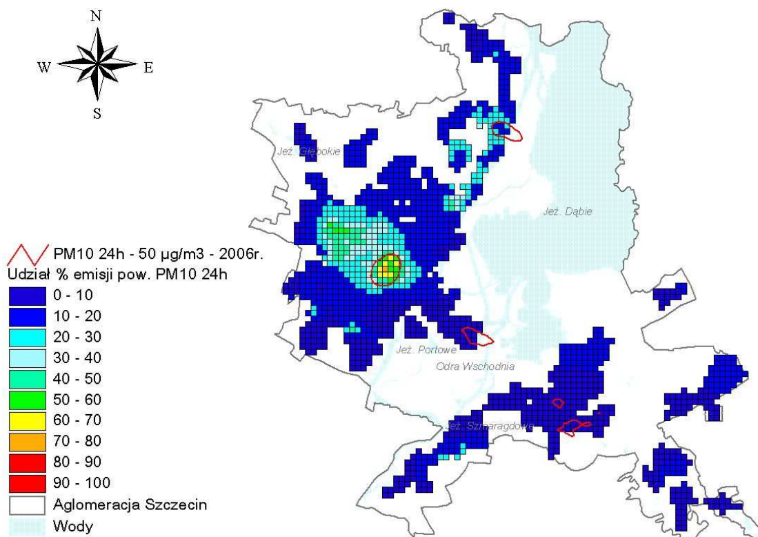
Rysunek 36 Procentowy udział emisji powierzchniowej w receptorach na obszarze aglomeracji Szczecin, w których w stężeniach pyłu zawieszzonego PM 10 24 godziny przeważa emisja powierzchniowa.
