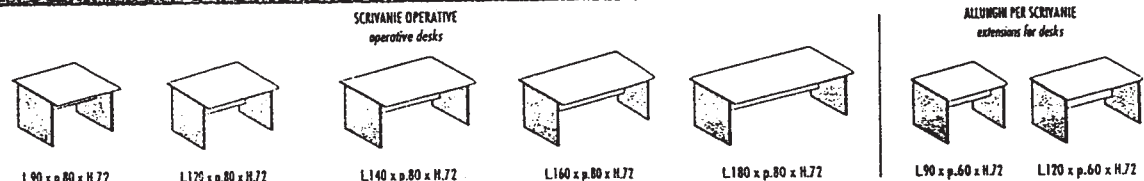
L90 x p.80 x H.72 L120 x p.80 x H.72 L140 x p.80 x H.72 L160 x p.80 x H.72 L180 x p.80 x H.72 L90 x p.60 x H.72 L120 x p.60 x H.72
