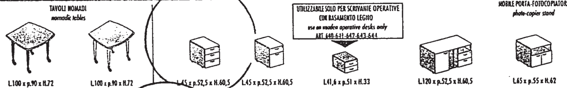
L100 x p.90 x H.72 L100 x p.90 x H.72 L45 x p.52,5 x H.60,5 L45 x p.52,5 x H.60,5 L41,6 x p.51 x H.33 L120 x p.52,5 x H.60,5 L45 x p.55 x H.62
