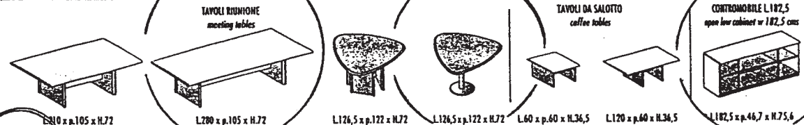
L110 x p.105 x H.72 L280 x p.105 x H.72 L126,5 x p.122 x H.72 L126,5 x p.122 x H.72 L60 x p.60 x H.34,5 L120 x p.60 x H.34,5 L182,5 x p.46,7 x H.75,6
