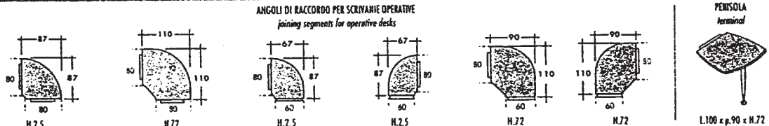
H.2,5 H.72 H.2,5 H.2,5 H.72 H.72 L100 x p.90 x H.72
