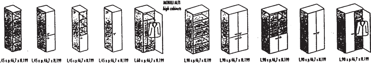
L45 x p.46,7 x H.199 L45 x p.46,7 x H.199 L45 x p.46,7 x H.199 L45 x p.46,7 x H.199 L60 x p.46,7 x H.199 L90 x p.46,7 x H.199 L90 x p.46,7 x H.199 L90 x p.46,7 x H.199 L90 x p.46,7 x H.199 L90 x p.46,7 x H.199
